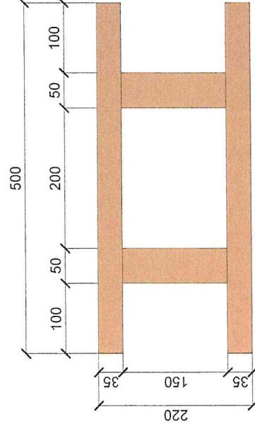
VISTA SUPERIORE
